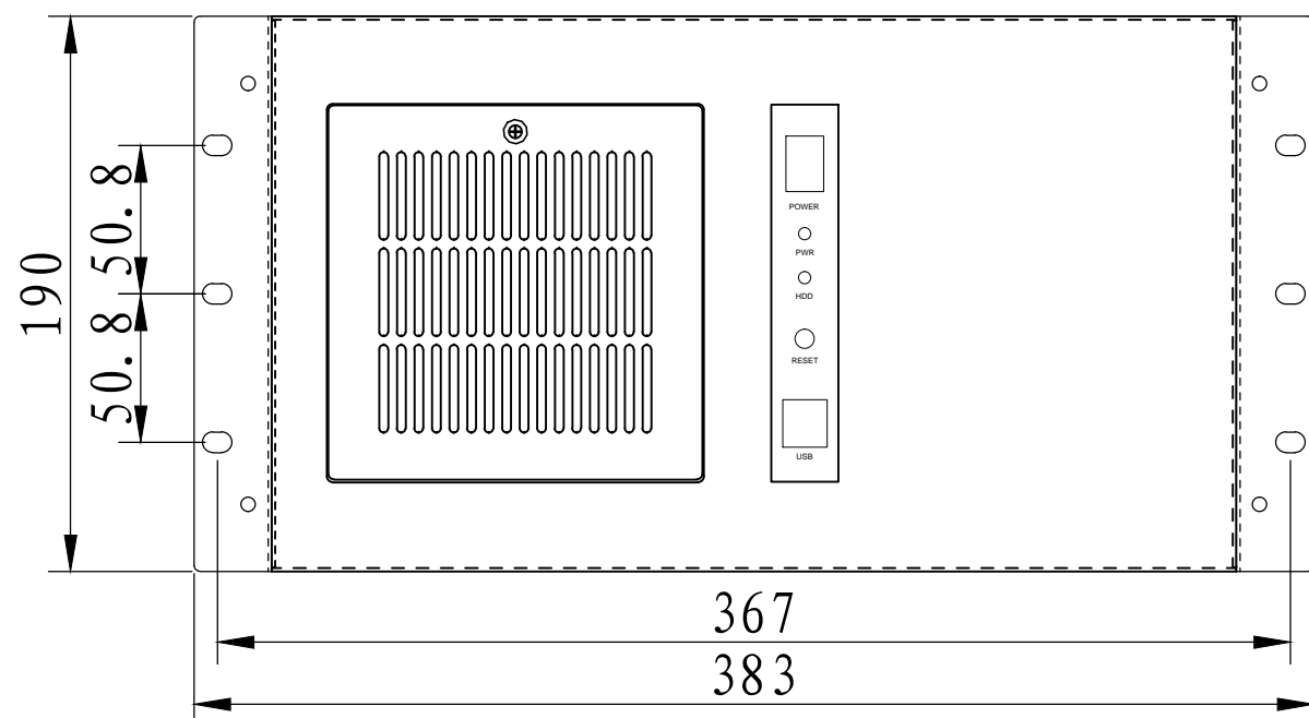
P向视图
