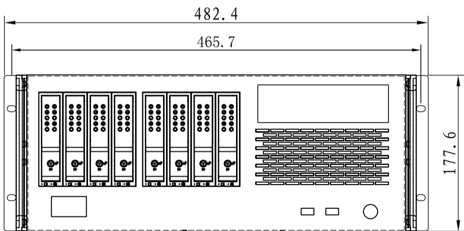
P向视图
