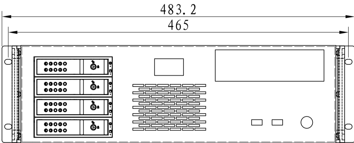
P向视图
