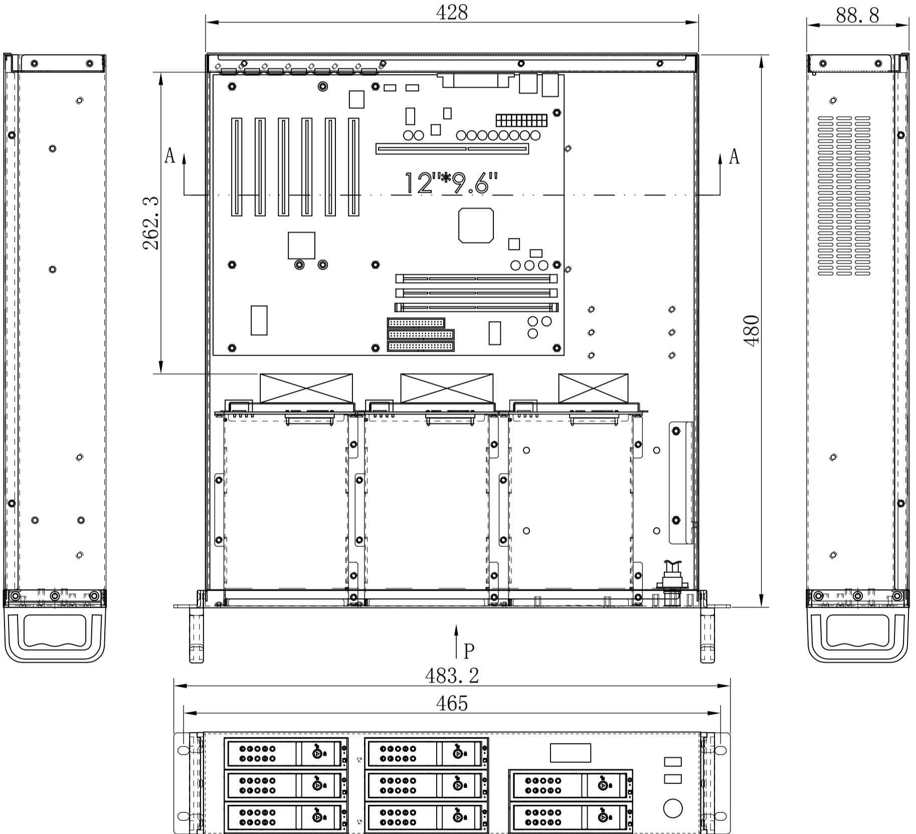
P向视图
