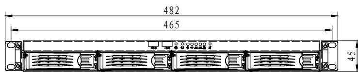
P向
