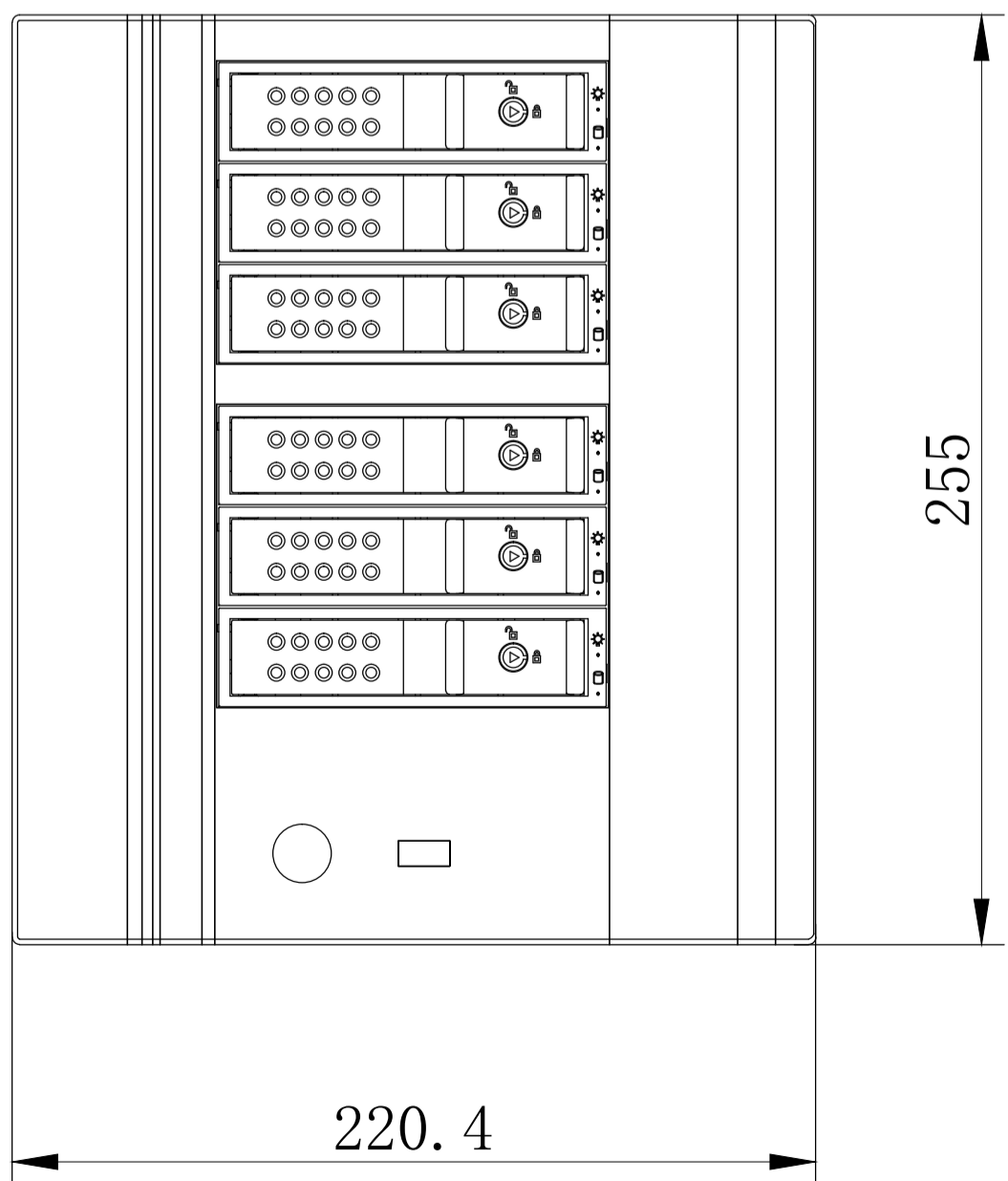
A向视图
