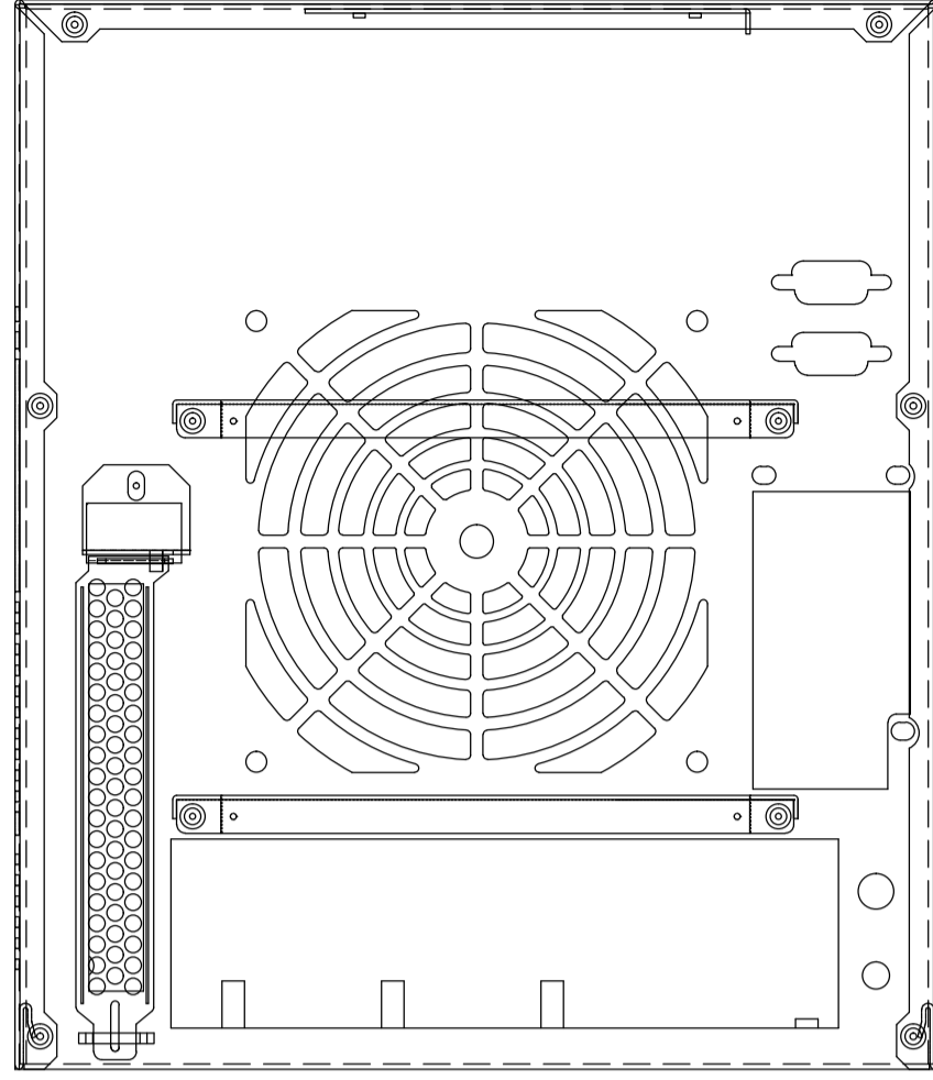
B-B
