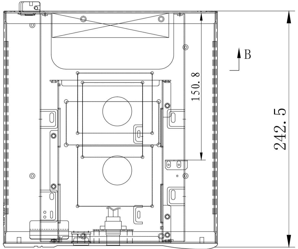
A向视图
