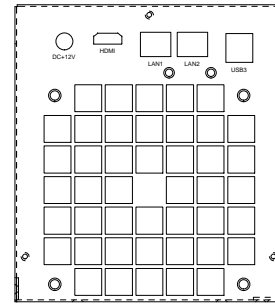
箱体后窗正面图
