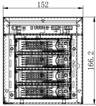
箱体正面图
