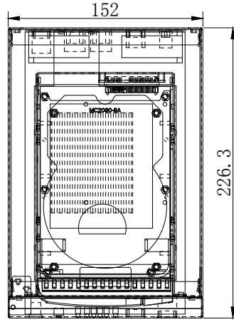
箱体正面图
