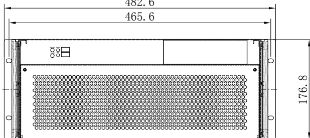
P向视图
