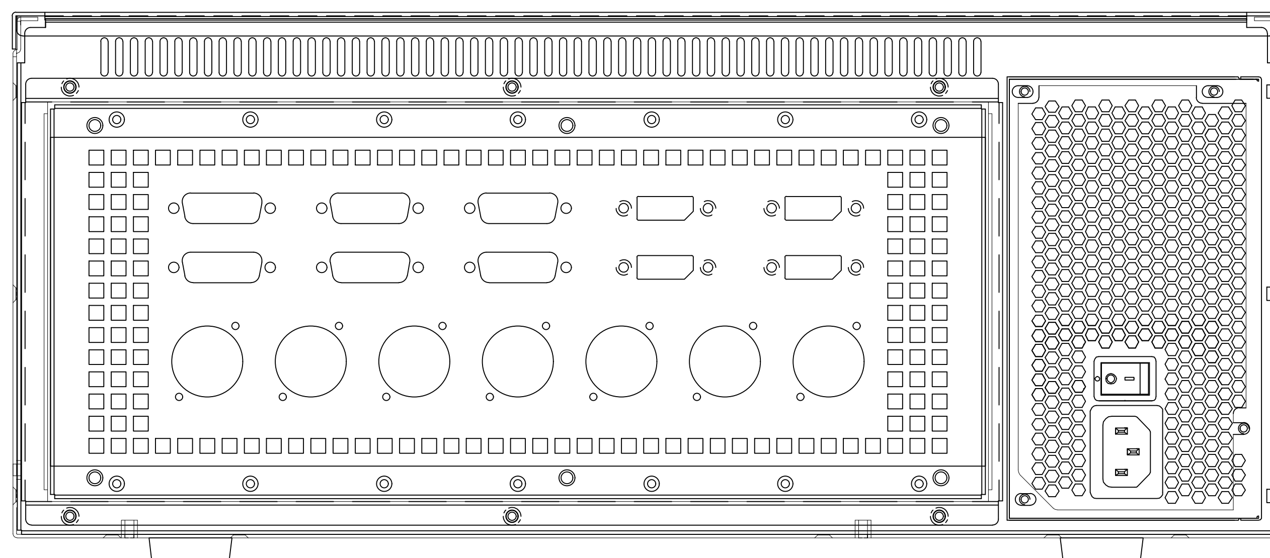
A-A A1款
