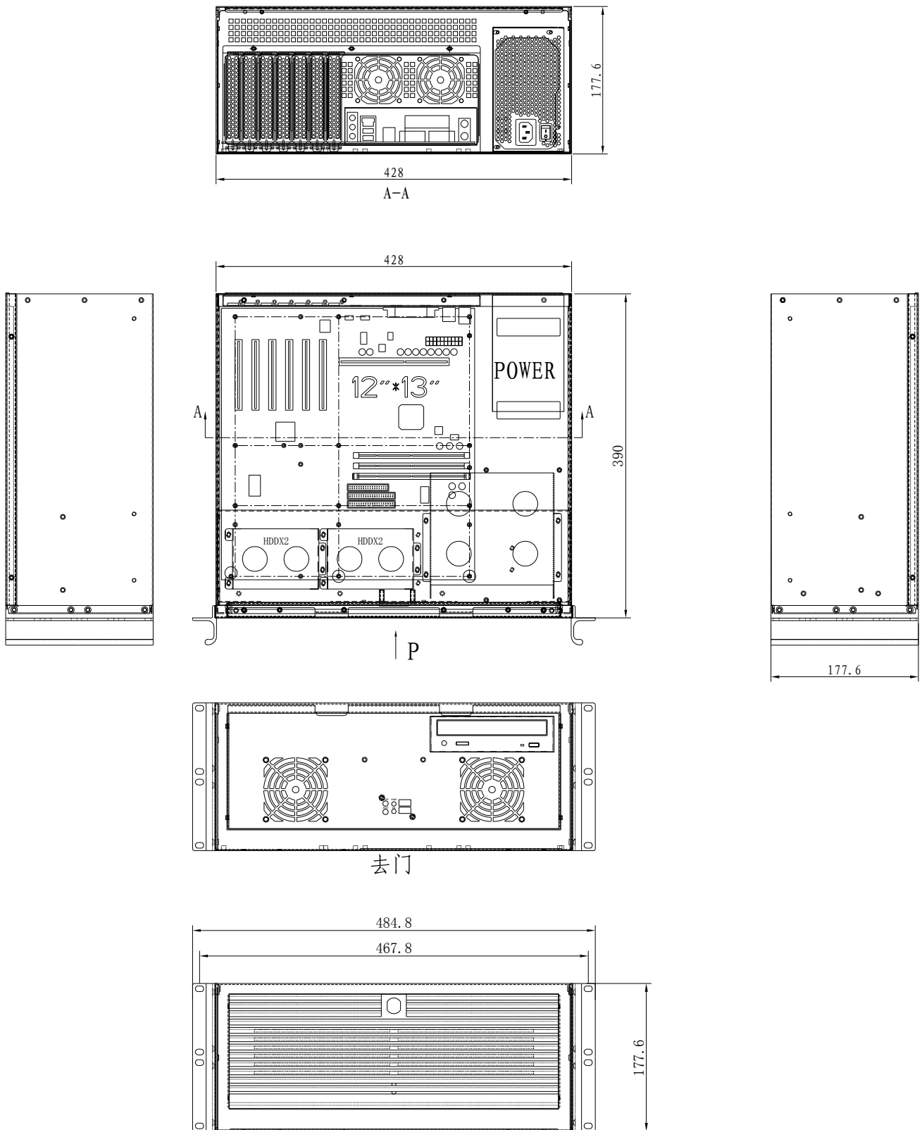
视图P
