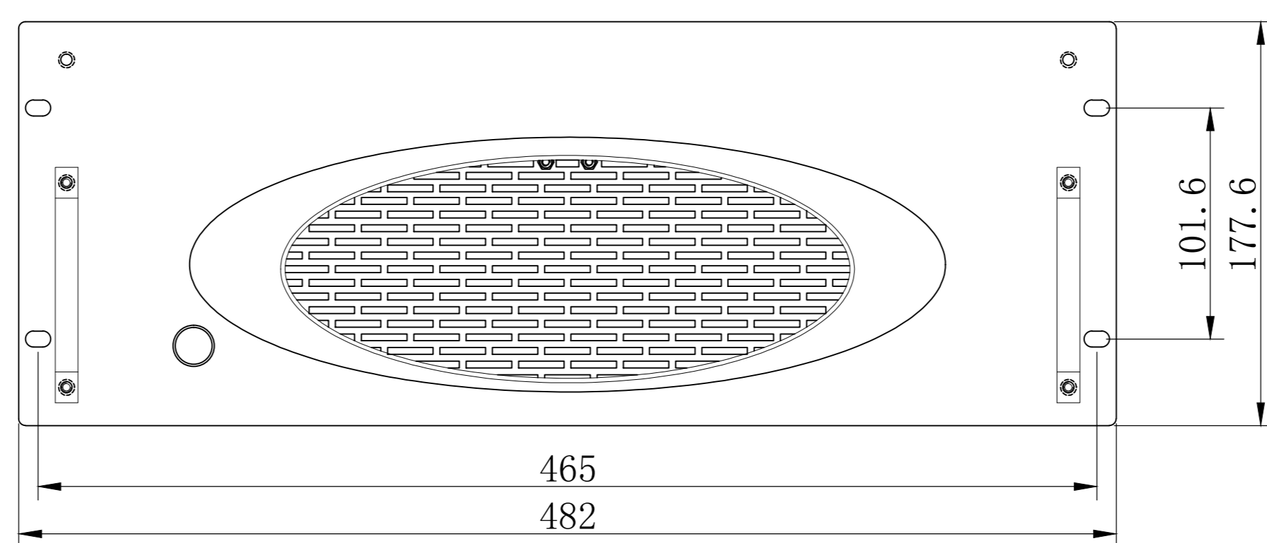
P向
