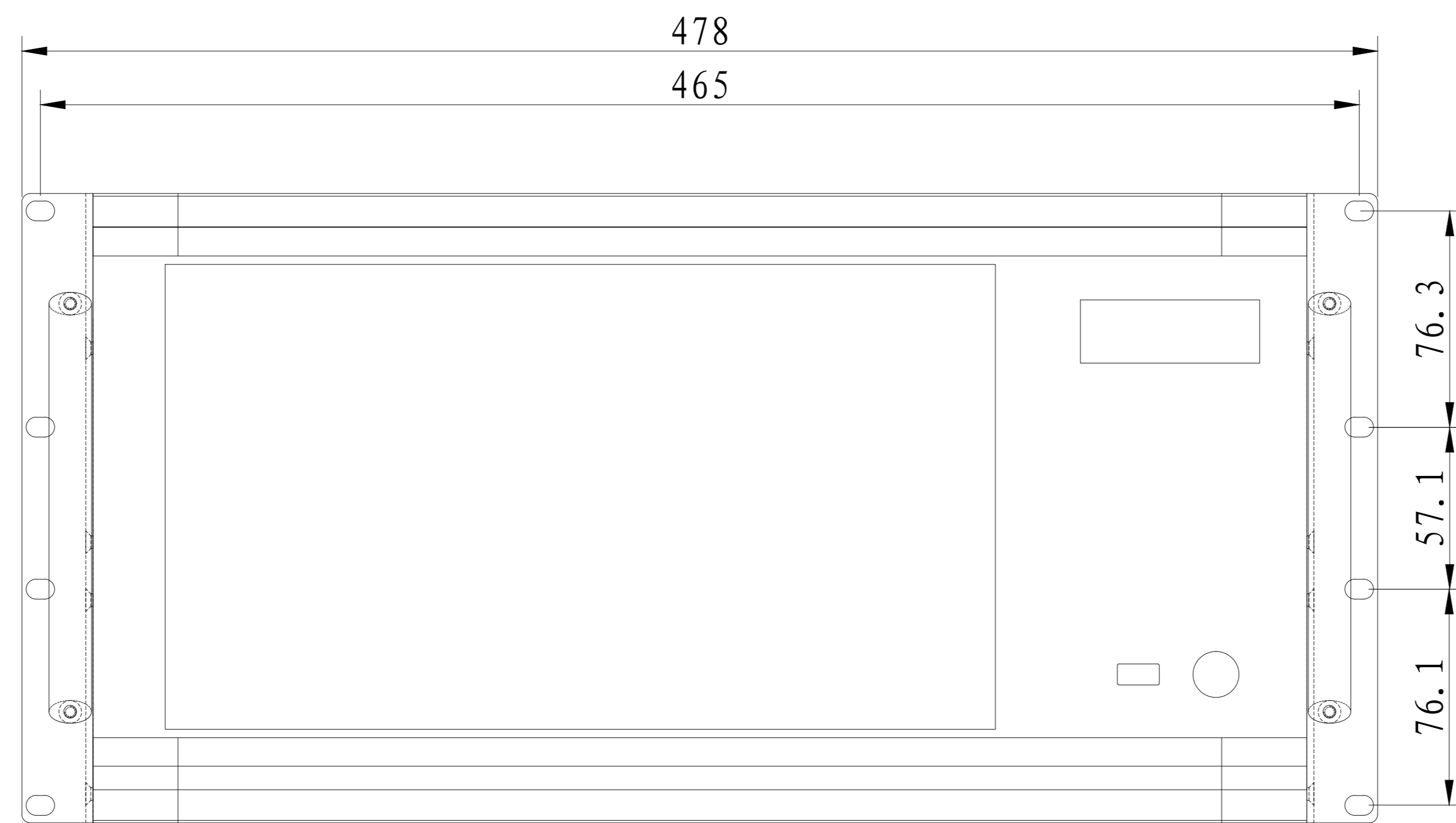
P向视图
